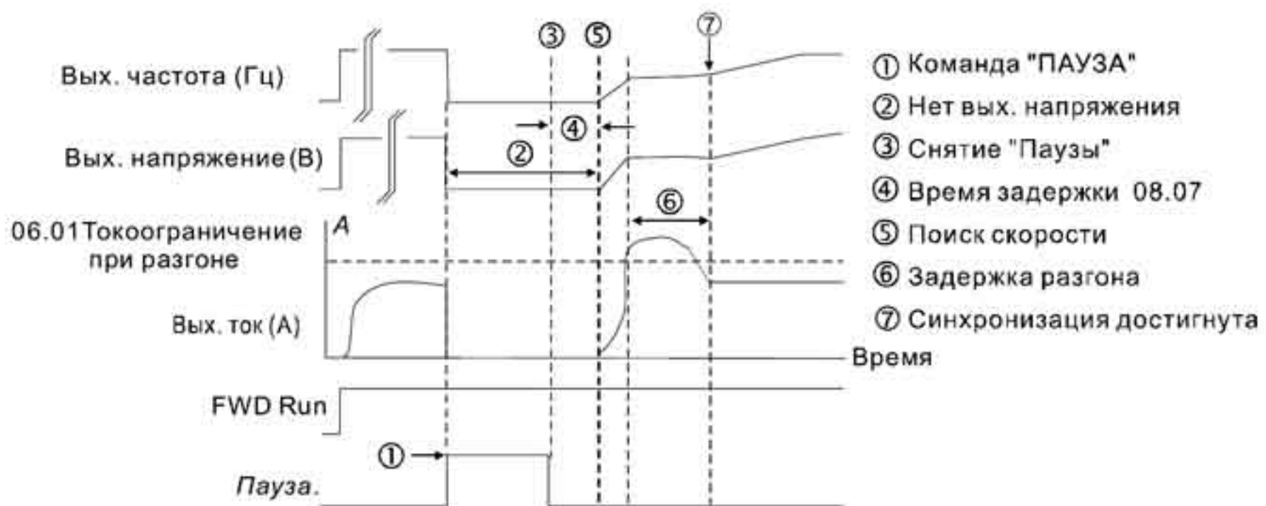
Рис 3: Поиск скорости с минимального значения частоты
