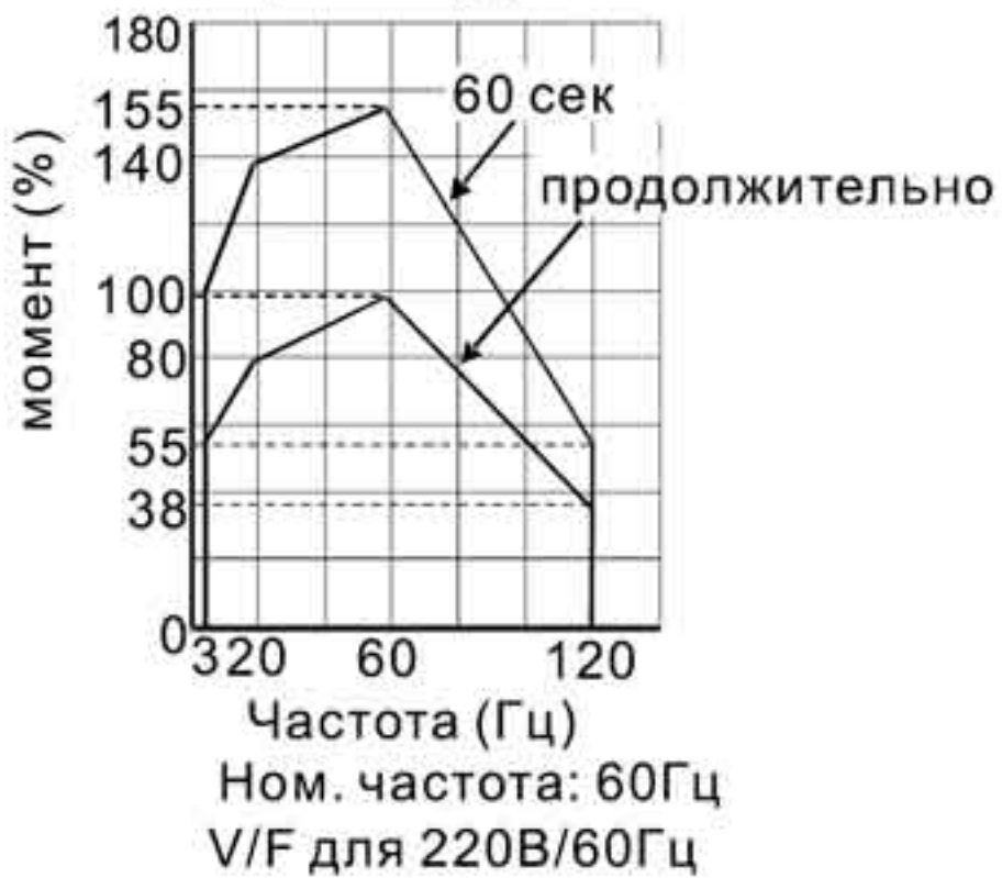
Асинхронный двигатель
